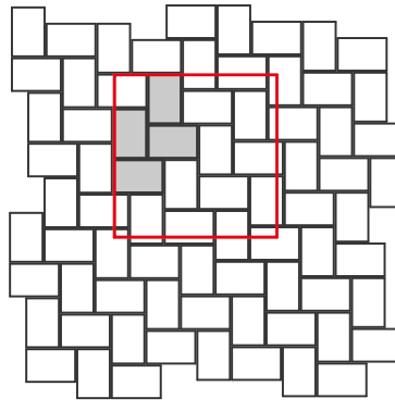
VM-28 26x15,6 (24,5 db/m 2 )
