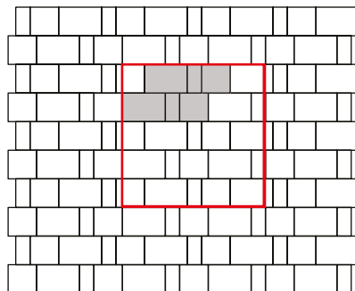
VM-18 30x20, 20x20, 20x10
