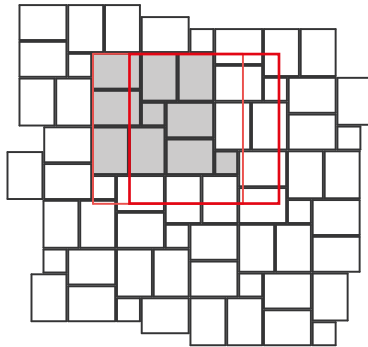
VM-21 32x24 (11,7 db/m 2 ), 16x16 (3,9 db/m 2 )
