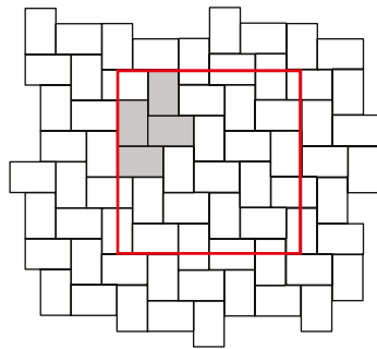
VM-12 30x20 (16,7 db/m 2 )
