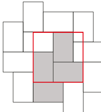
VM-34 60x40 (4,2 db/m 2 )
