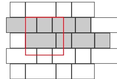
VM-03 80x40 (1,1 db/m 2 ), 60x40 (1,1 db/m 2 ), 40x40 (2,3 db/m 2 )
