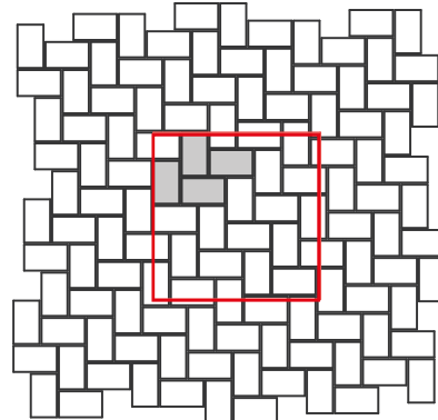
VM-29 26x15,6 (24,5 db/m 2 )
