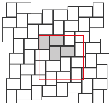
VM-20 32x24 (12,8 db/m 2 )
